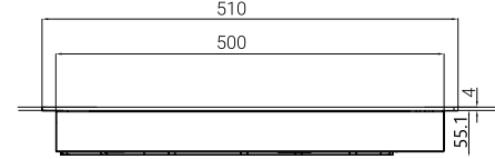
Önden Görünüş
