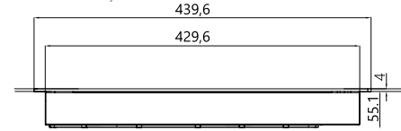
Önden Görünüş
