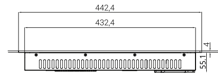
Yan Görünüm
